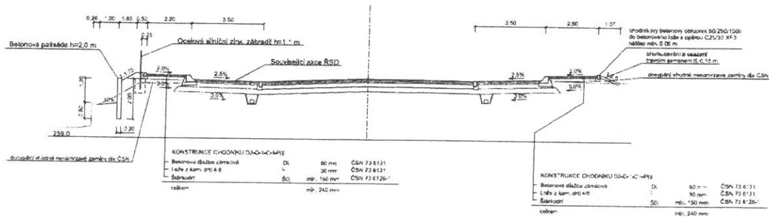
VZOROVÝ PŘÍČNÝ ŘEZ M 1:100
