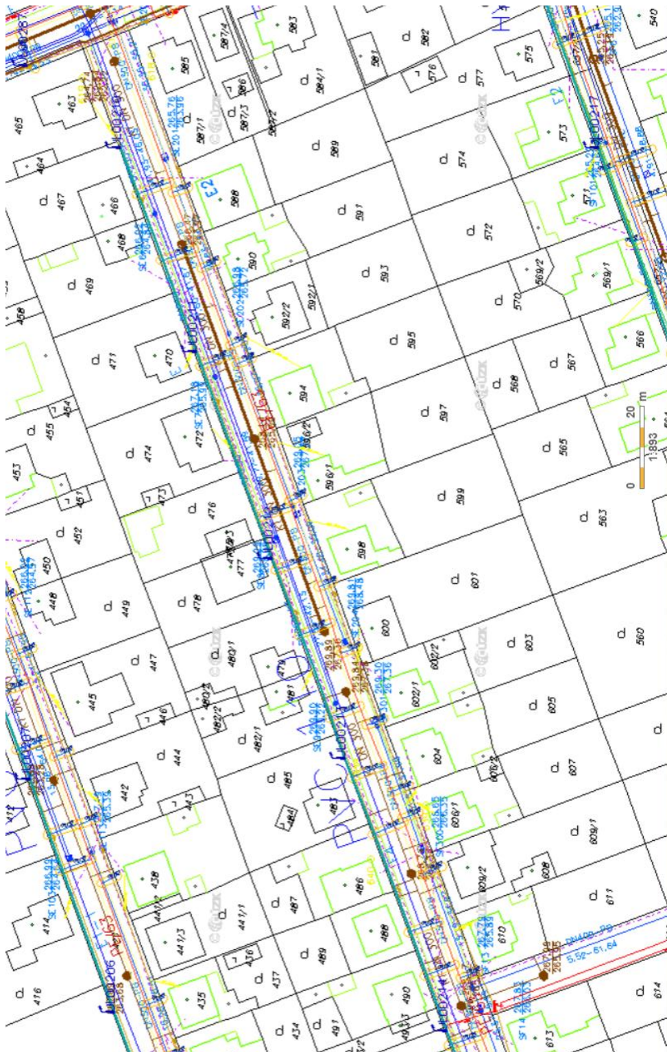
Převzatý záměr ing. sítí z technické mapy města Úvaly – detailněji viz https://uvaly.obce.gepro.cz/#/
